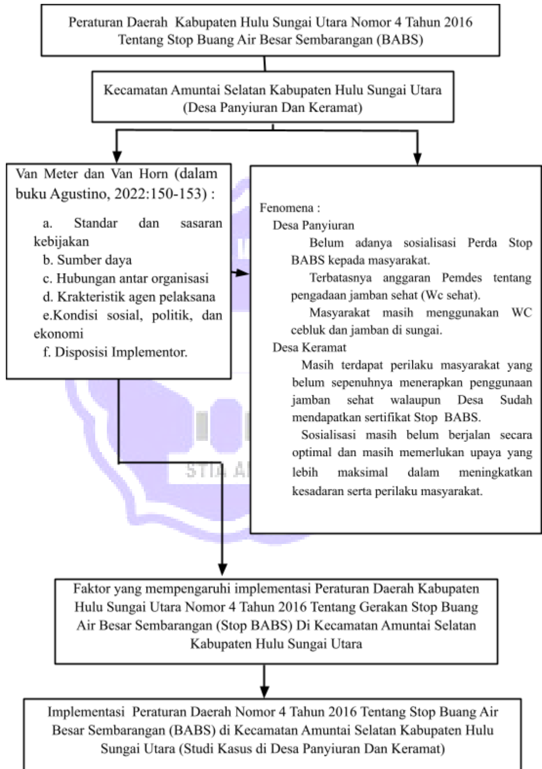
Gambar 2.2 Kerangka Pemikiran
