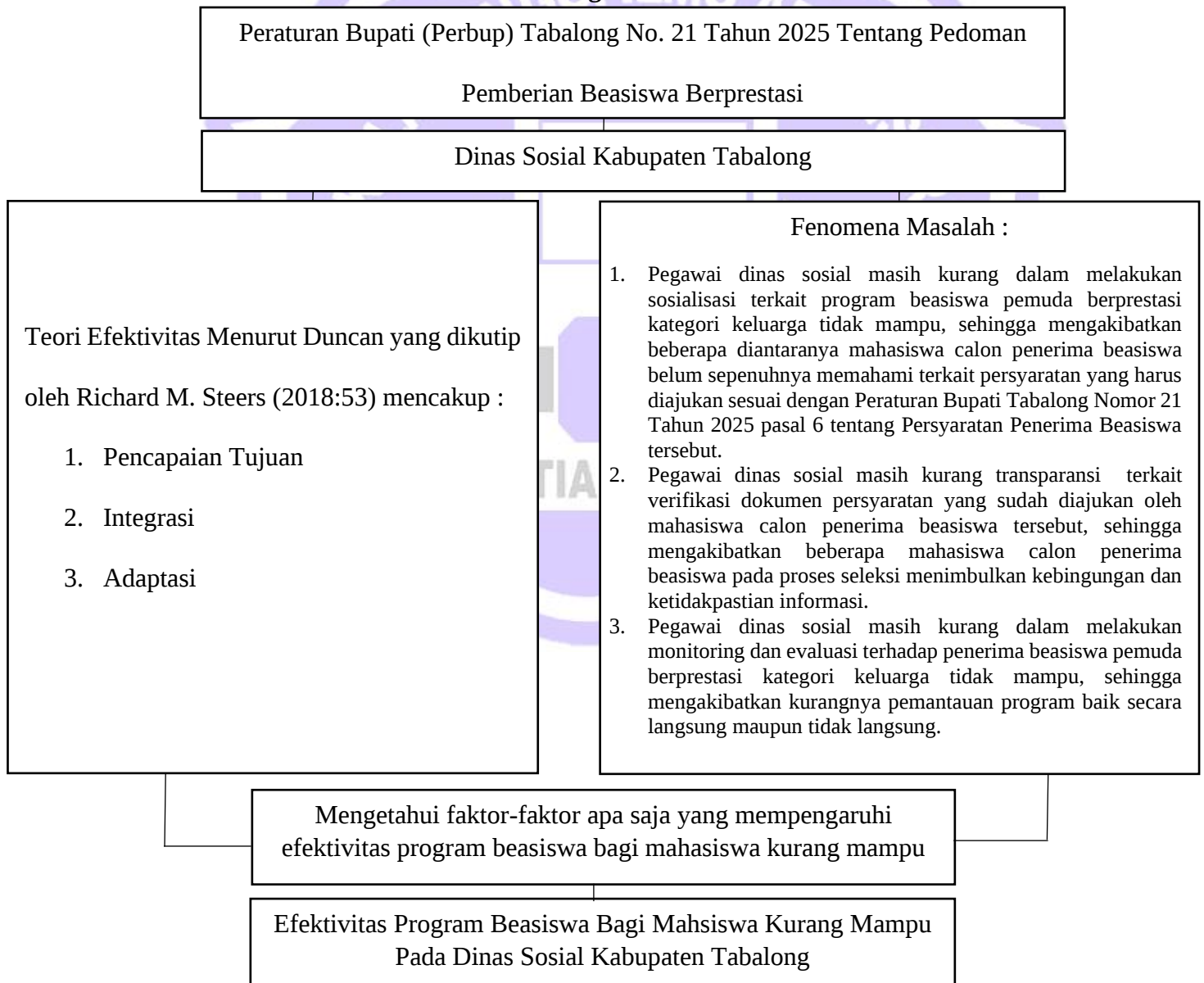
Gambar 2.1 Kerangka Pemikiran
