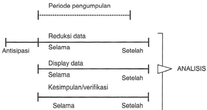
Gambar 13.1a. Komponen dalam analisis data ( flow model )
