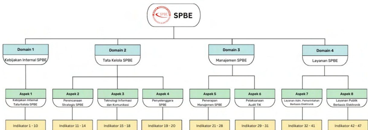
Gambar 5. Struktur Penilaian Tingkat Kematangan SPBE
